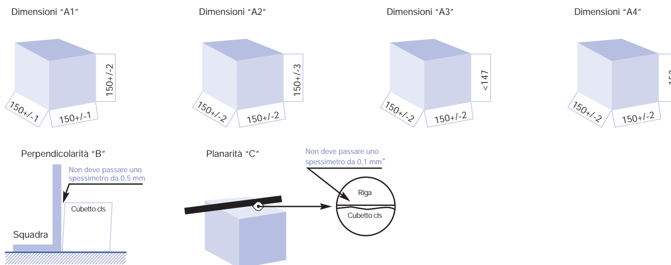
Verifiche dimensionali sui cubetti di calcestruzzo
